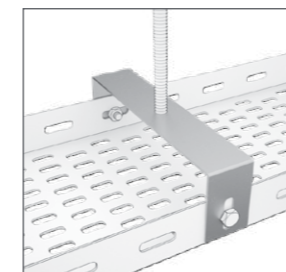
Support atârnare jgheab cu diferite dimensiuni / Single rod tray carriers
