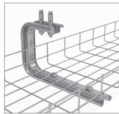
Etrier suspendat jgheab / C bracket
