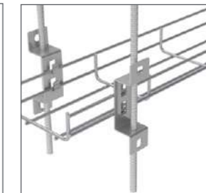
Piesă suspendare jgheab sârmă / Bracket for wall and floor mounting
